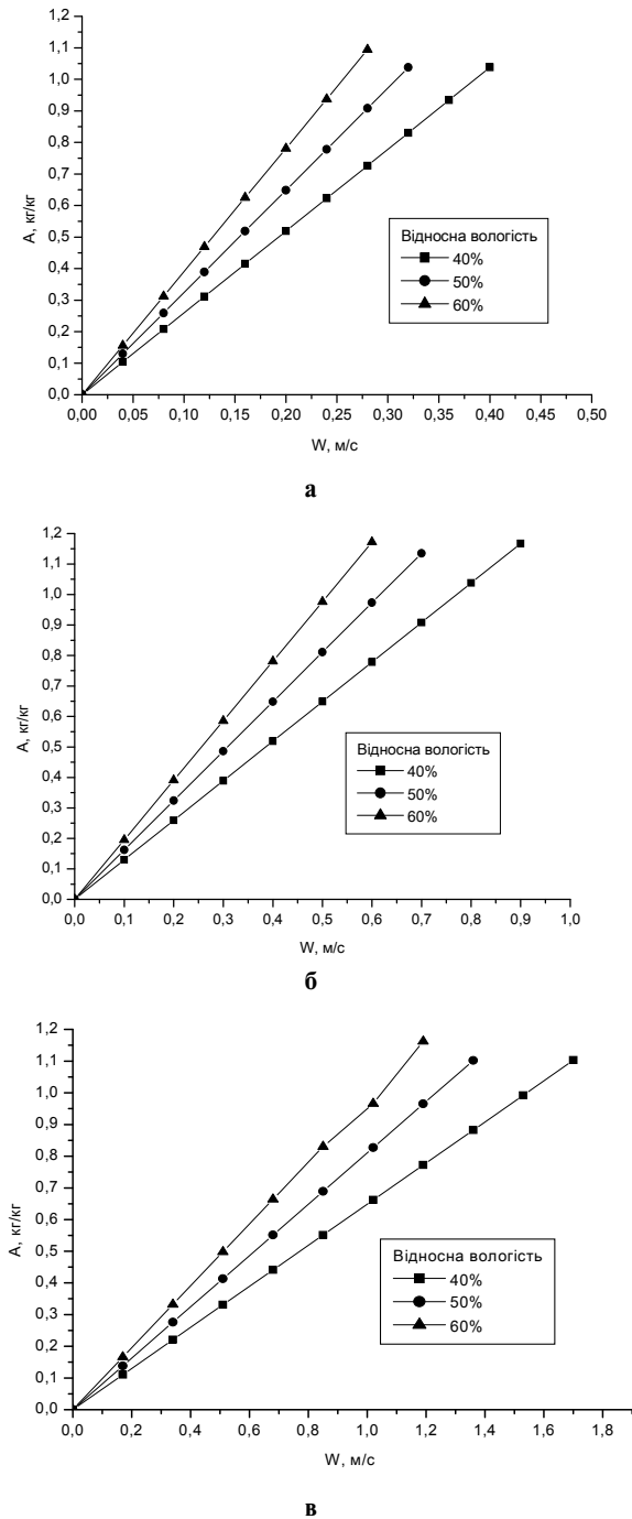
Рис. 3. Залежність величини сорбції від швидкості пароговзного потоку та висоти шару композиту та відносній вологості повітря: а – H=0,25 м; б – H=0,5 м; в – H=1 м
